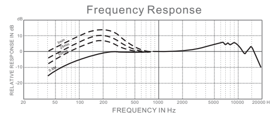
PRO248/PRO248S 典型頻率響應(圖2)
