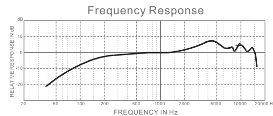
PRO258 典型頻率響應(圖4)
