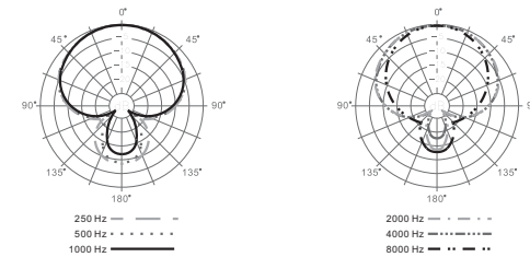
PRO248/PRO248S 典型的超心型極座標圖型(圖1)
