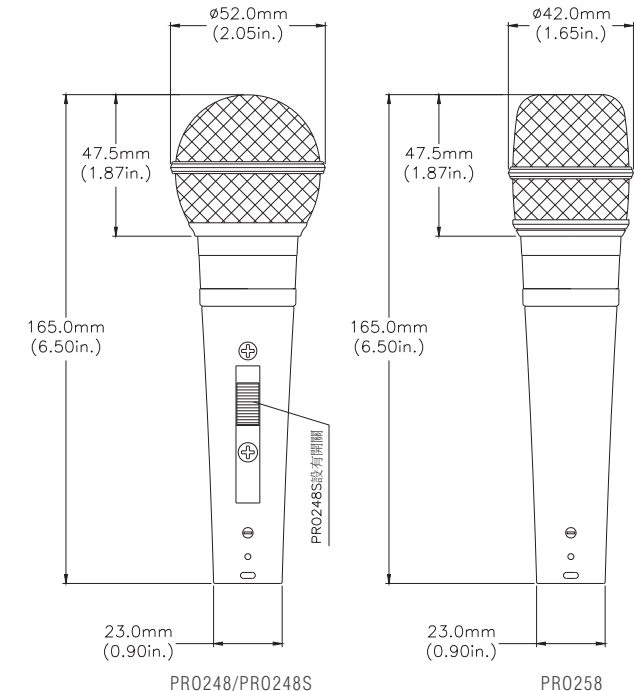
外型尺寸圖(圖5)
