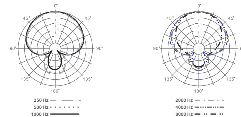
PRO258 典型的超心型極座標圖型(圖3)
