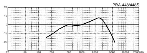
频率响应
