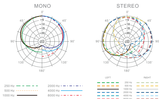
E523D 频率响应图 (心型)
