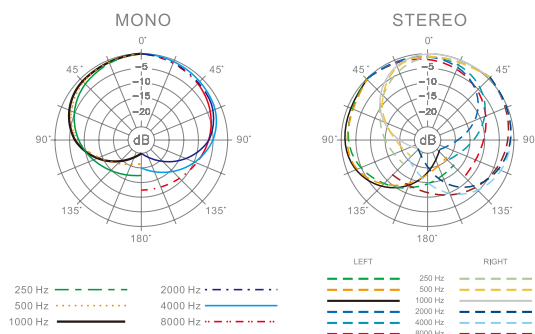
E523D 頻率響應圖 (心型)
