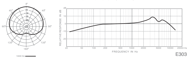
E303 频率响应图 (心型)
