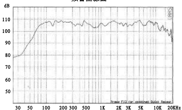
頻響曲線圖
