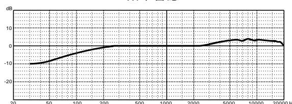
頻率響應
