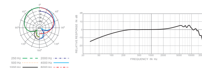
D10D 频率响应图 (超心型)
