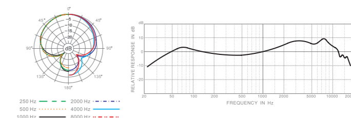
PRA218B 頻率響應圖（超心型）
