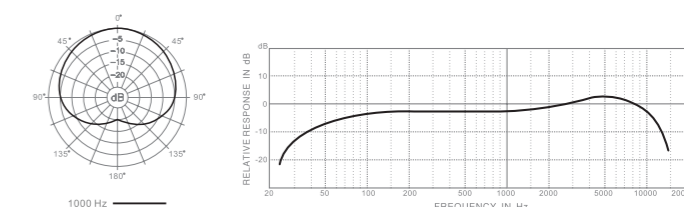
E102 頻率響應圖（心型）
