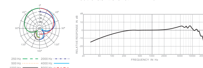
D10D 頻率響應圖（超心型）
