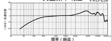
典型频率响应 PRO-258
