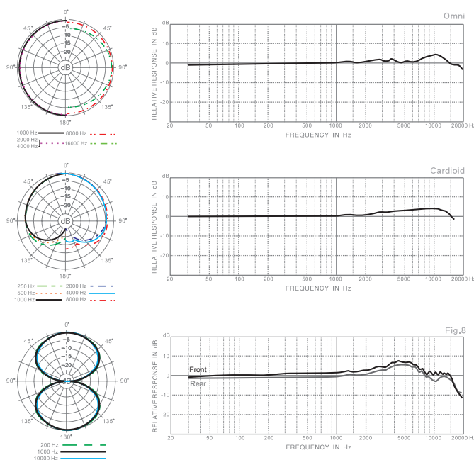
CMH8G 频率响应图
