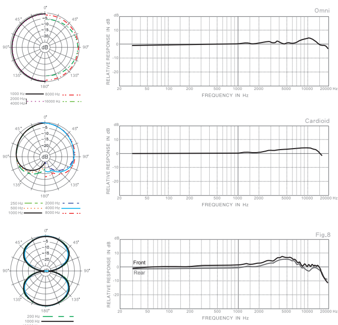
CMH8G 頻率響應圖
