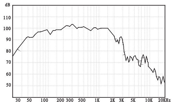
頻響曲線圖
