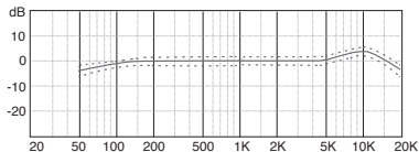
S502MKII 頻率響應圖 (心型)
