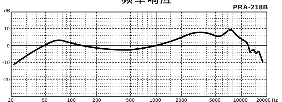
频率响应
