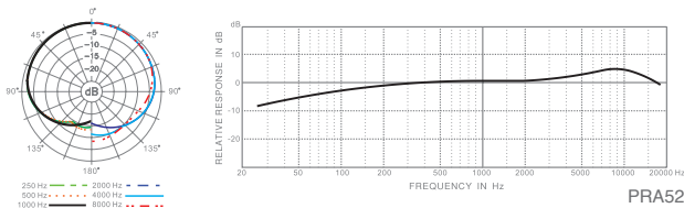
PRA52 频率响应图 (心型)
