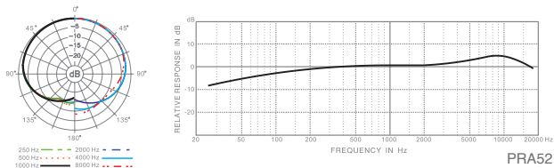
PRA52 頻率響應圖 (心型)
