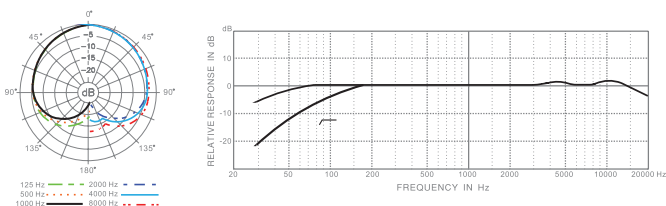
CMH8B 频率响应图
