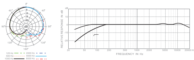
CMH8B 頻率響應圖
