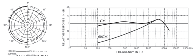
PRA535NC 頻率響應圖
