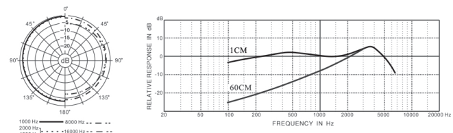
PRA535NC 频率响应图
