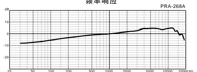
频率响应
