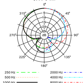
指向性
