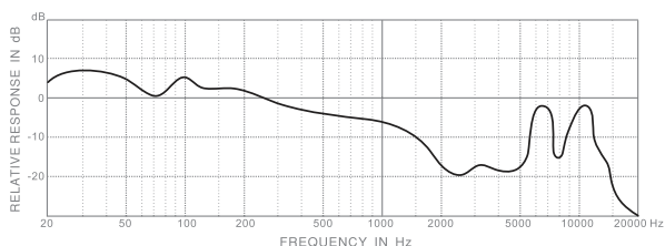
HMC631 频率响应图 (心型)
