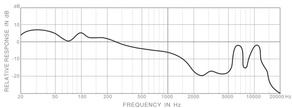
HMC631 頻率響應圖（心型）
