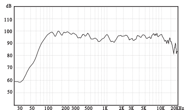
频率响应图
