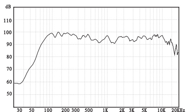
頻響曲線圖
