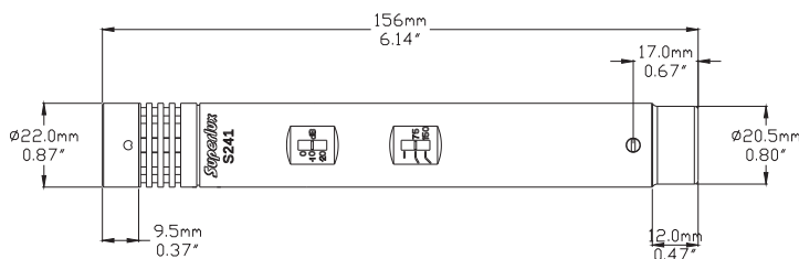
外观尺寸图
