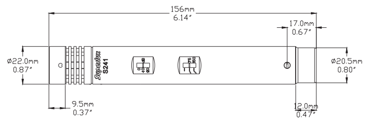
外觀尺寸圖
