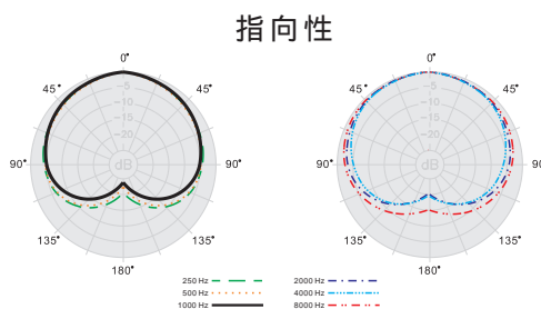
指向性
