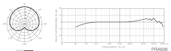
PRA638 频率响应图 (心型)
