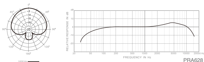
PRA628 频率响应图 (超心型)
