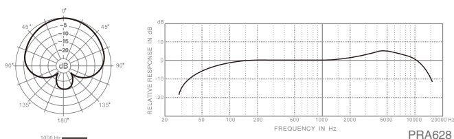
PRA628 頻率響應圖 (超心型)
