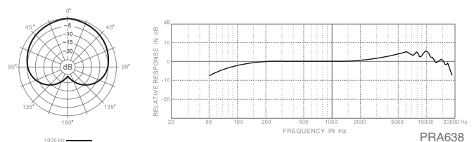
PRA638 頻率響應圖 (心型)
