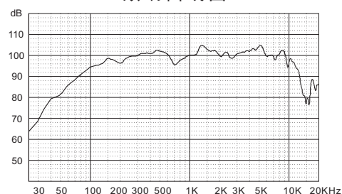
频响曲线图
