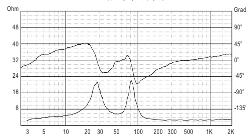
阻抗曲线图
