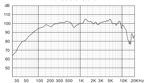
頻響曲線圖
