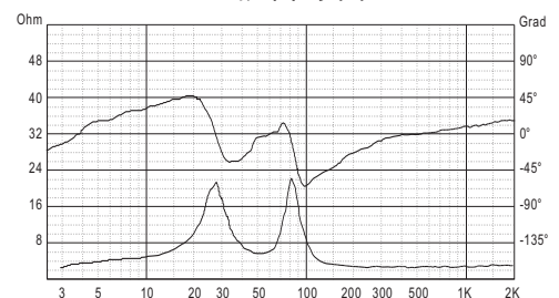
阻抗曲線圖
