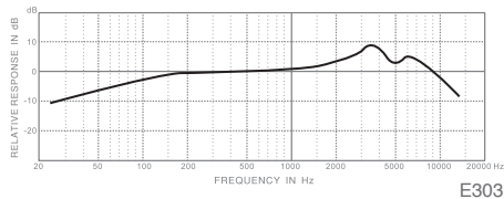
E303 頻率響應圖 (心型)
