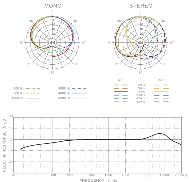
E524D 频率响应图 (心型)
