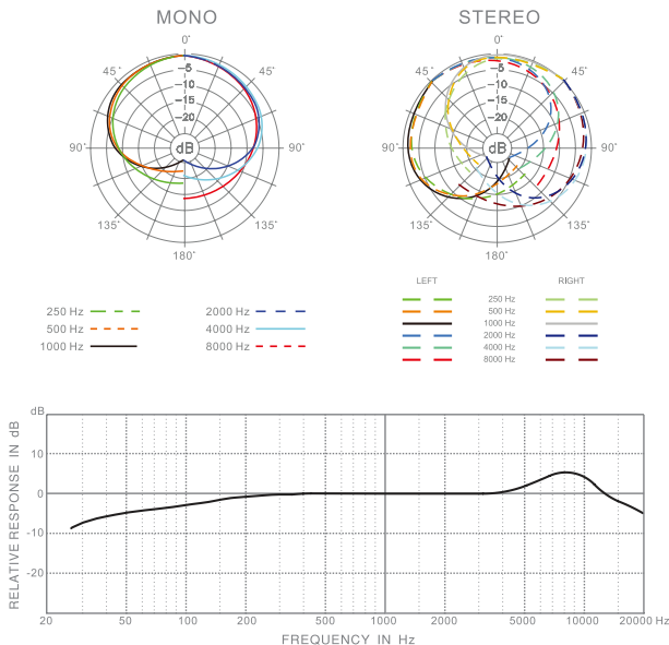
E524D 頻率響應圖（心型）
