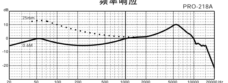
频率响应
