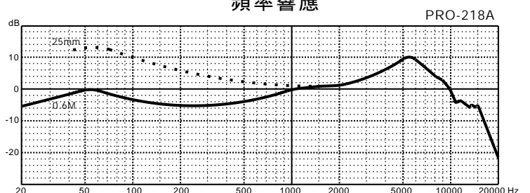
頻率響應
