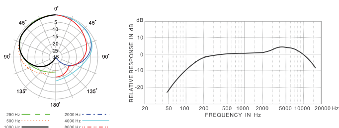
HMD660 频率响应图 (心型)
