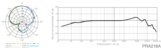
PRA218A 頻率響應圖（超心型）
