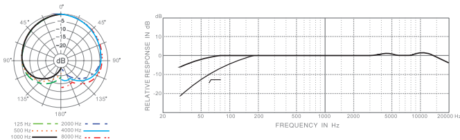
CMH8A 频率响应图
