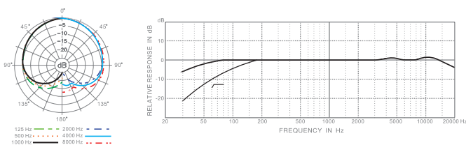
CMH8A 頻率響應圖
