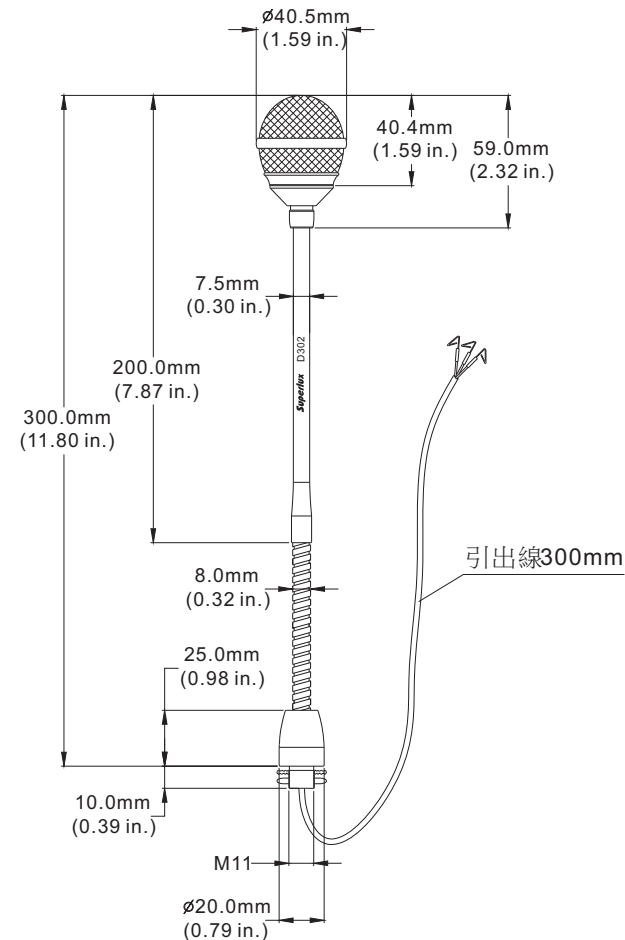
外型尺寸圖(圖3)
