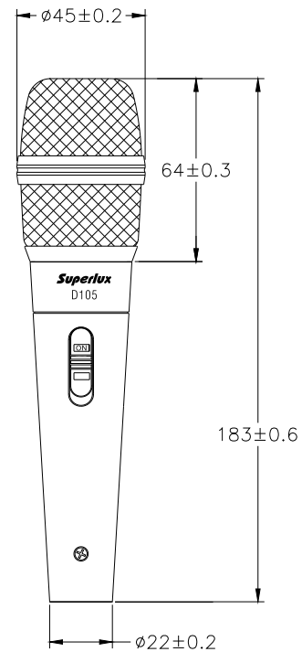
外型尺寸(图3)
