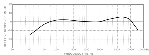
频率响应 (图2)
