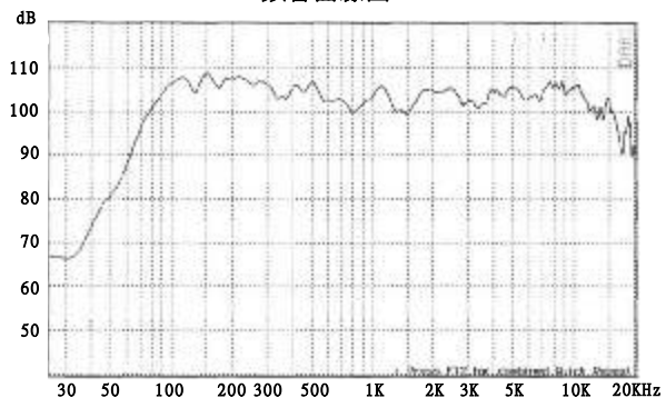
頻響曲線圖
