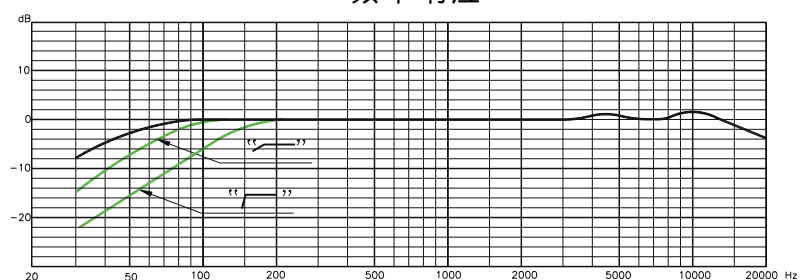
频率响应
