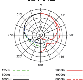
指向性
