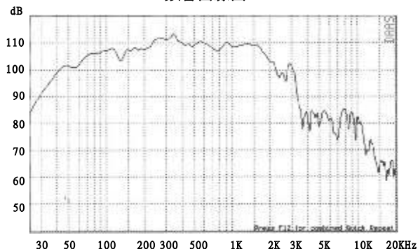
頻響曲線圖
