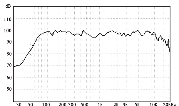
頻響曲線圖
