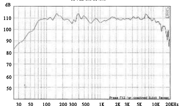
頻響曲線圖
