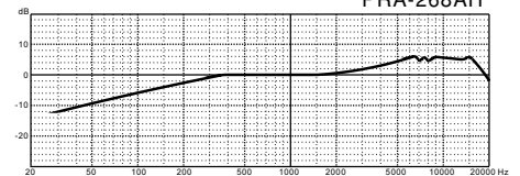
頻率響應 PRA-268AH
