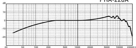
頻率響應 PRA-228A
