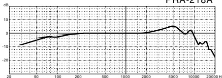
頻率響應 PRA-218A
