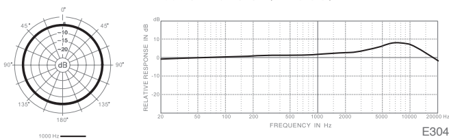
E304 频率响应图 (无指向)
