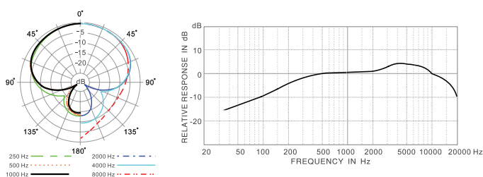
HMC660 频率响应图 (超心型)
